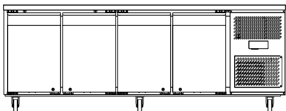
4 x Solid Doors AXR.UCGN.4 2230 x 700 x 840
